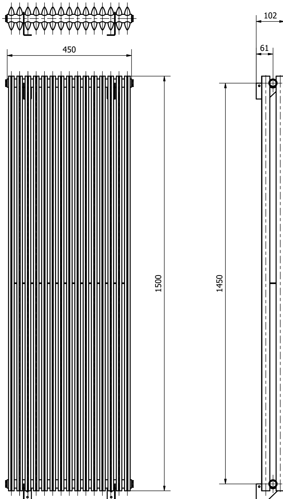
LUXRAD Aurora Podwójna 1500x450
